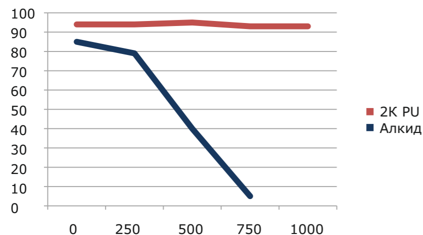
Испытания на светостойкость в аппарате искусственной погоды QUV UVA 340
